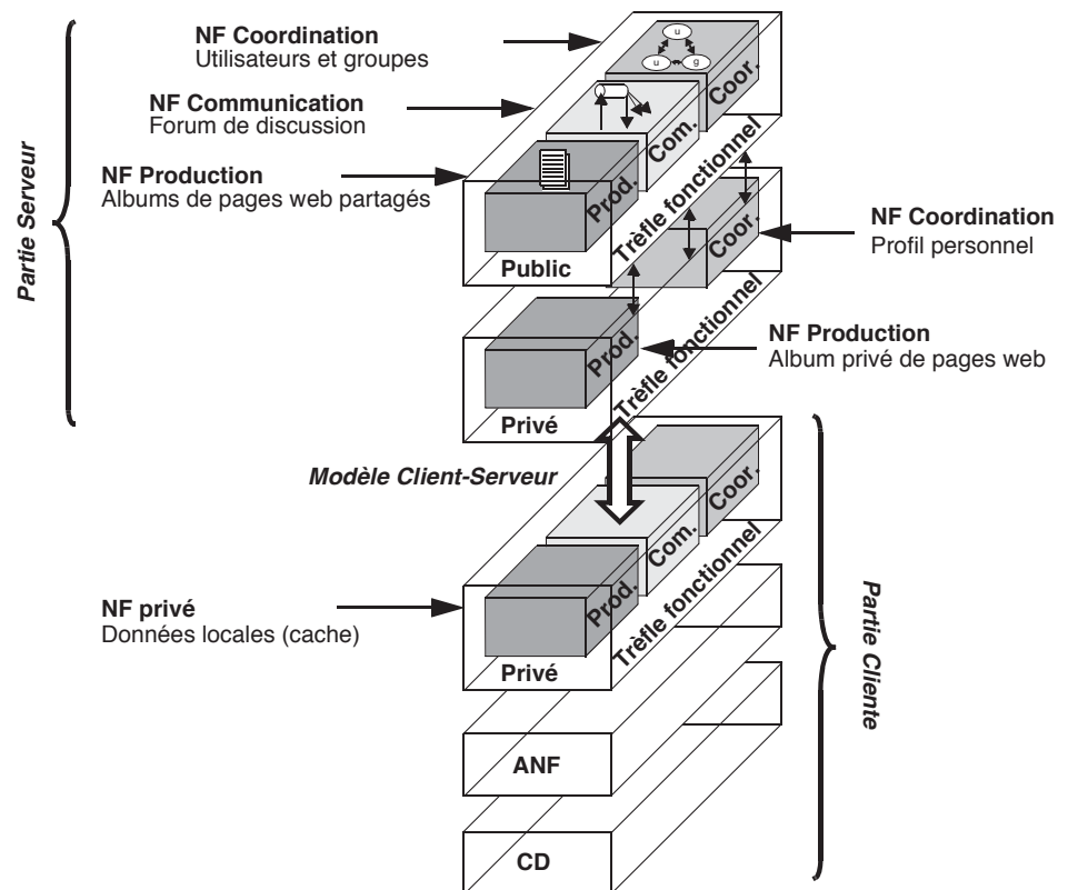
Figure 13 Architecture de CoVitesse selon le modèle Clover
