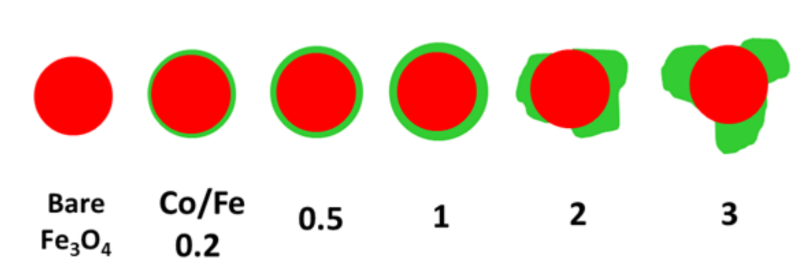
Figure 3: Représentation schématisée des NPs cœur-coquille \text{Fe}_3\text{O}_4@\text{CoO} (CoO -coquille, en vert et cœur de \text{Fe}_3\text{O}_4 en rouge) en fonction du rapport molaire Co /Fe.
