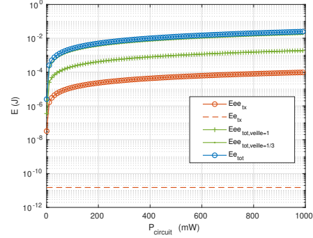
FIGURE 1 – Énergie transmise et totale en fonction de P_{\text{circuit}} .
