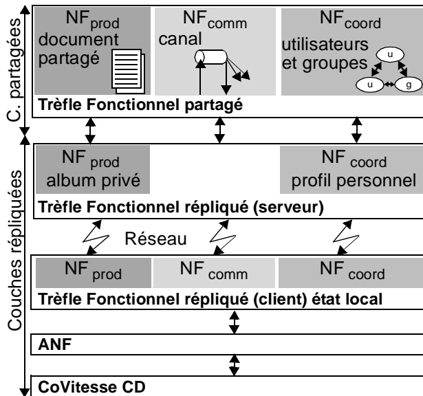
Figure 7: Architecture implémentationnelle de CoVitesse.
