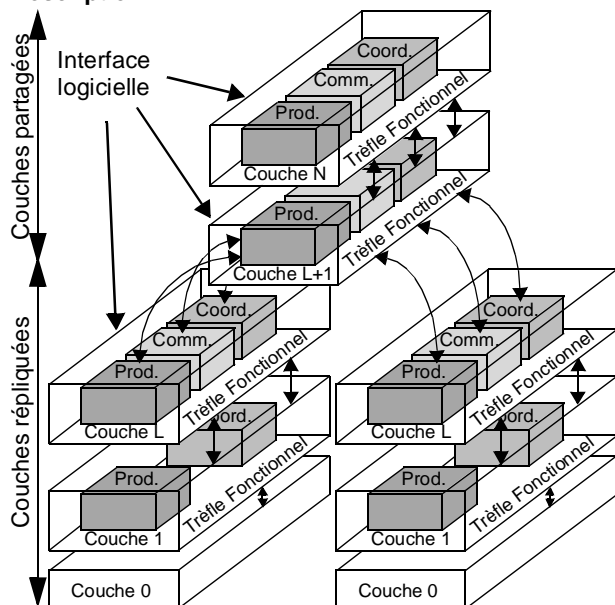
Figure 6: Métamodèle d'architecture Clover.
