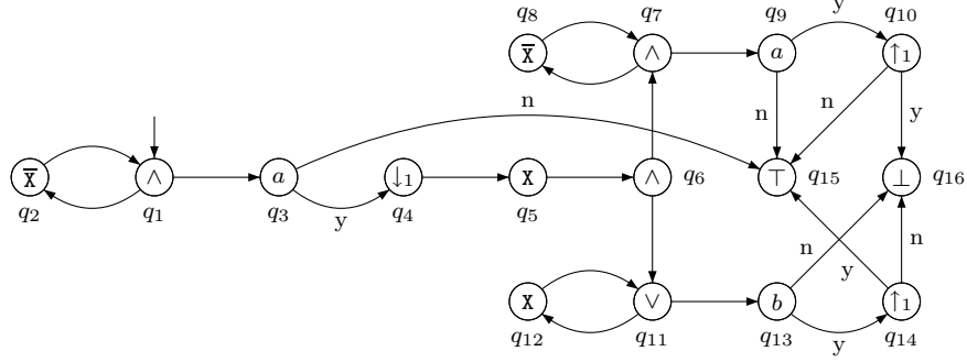
Fig. 3. A register automaton
