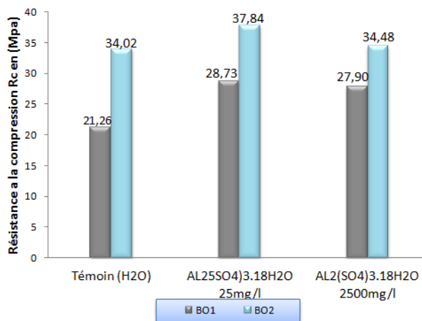
Figure 3. Variation de la résistance en compression.
