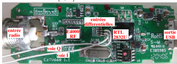
FIGURE 5 – Modifications matérielles sur récepteur DVB-T afin d'exploiter directement le convertisseur analogique-numérique sans passer par l'étage de démodulation radiofréquence.
