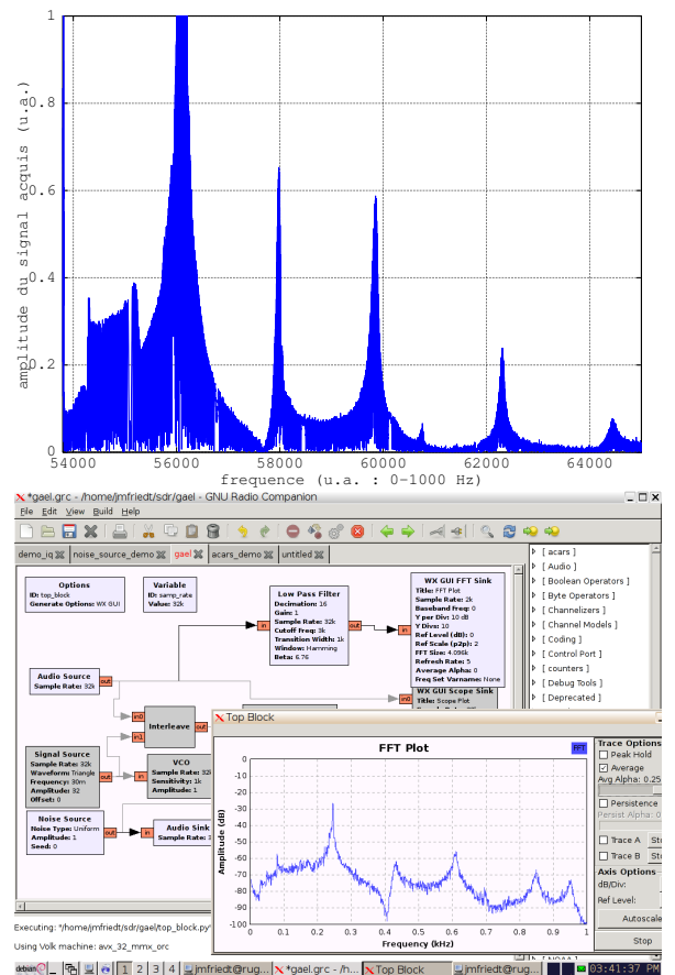
FIGURE 4 – Exemple de mesure acquise par une excitation par un bruit blanc du pot vibrant (en haut) et par balayage de fréquence (en bas). Les divers modes propres entre 0 et 1000 Hz sont clairement visibles.
