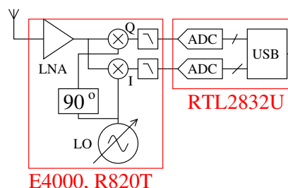
FIGURE 1 – Architecture du récepteur DVB-T : un démodulateur I/Q sans fréquence intermédiaire convertit le signal radiofréquence reçu par l'antenne après amplification (LNA – Low Noise Amplifier ) en signal basse-fréquence après mélange avec un oscillateur local (LO – Local Oscillator ) de fréquence configurable numériquement. L'Elonics
