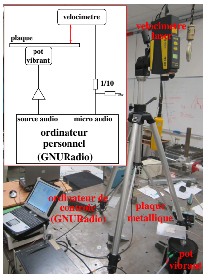
FIGURE 3 – Dispositif expérimental de mesure des modes propres d’une plaque vibrante.
