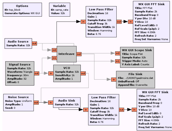
FIGURE 2 – Deux modes de fonctionnement d’analyseurs de réseaux audiofréquences sont présentés dans cette interface : en gris (commenté) un mode par balayage de fréquence dans lequel la réponse aux sollicitations successives par des signaux de fréquences variables est enregistrée ; et en couleur (actif) un mode par transformée de Fourier de la réponse excitée par une source de bruit blanc.
