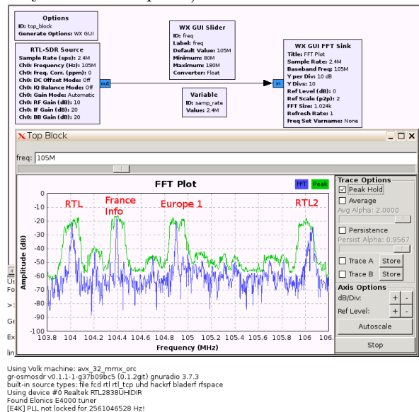
FIGURE 7 – Utilisation du récepteur de télévision numérique terrestre (DVB-T) comme analyseur de spectre dans la bande FM.
