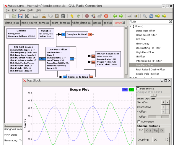
FIGURE 6 – Utilisation du convertisseur analogique-numérique d'un récepteur DVB-T pour échantillonner deux signaux, l'un sinusoïdal d'amplitude 150 mV pp , l'autre triangulaire d'amplitude 200 mV pp , tous deux de fréquence 40 kHz. Le filtre passe-bas a pour vocation d'illustrer la décimation entre la source et le puits.
