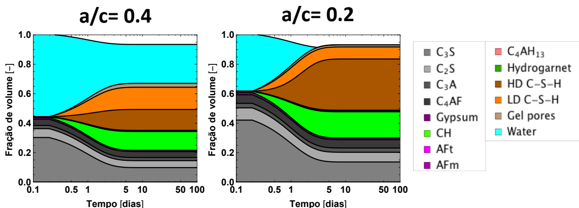
Figura 1 – Evolução das frações de volume das fases para um sistema com a/c inicial de 0.4 e 0.2
