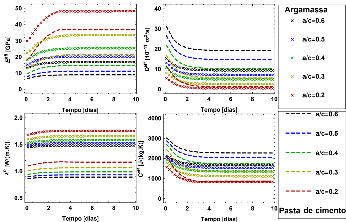
Figura 2 – Propriedades efetivas: modulo de elasticidade E^{eff} , condutividade térmica \lambda^{eff} , capacidade térmica C^{eff} e difusividade D^{eff} nas escalas da pasta de cimento (linhas) e da argamassa (símbolos).
