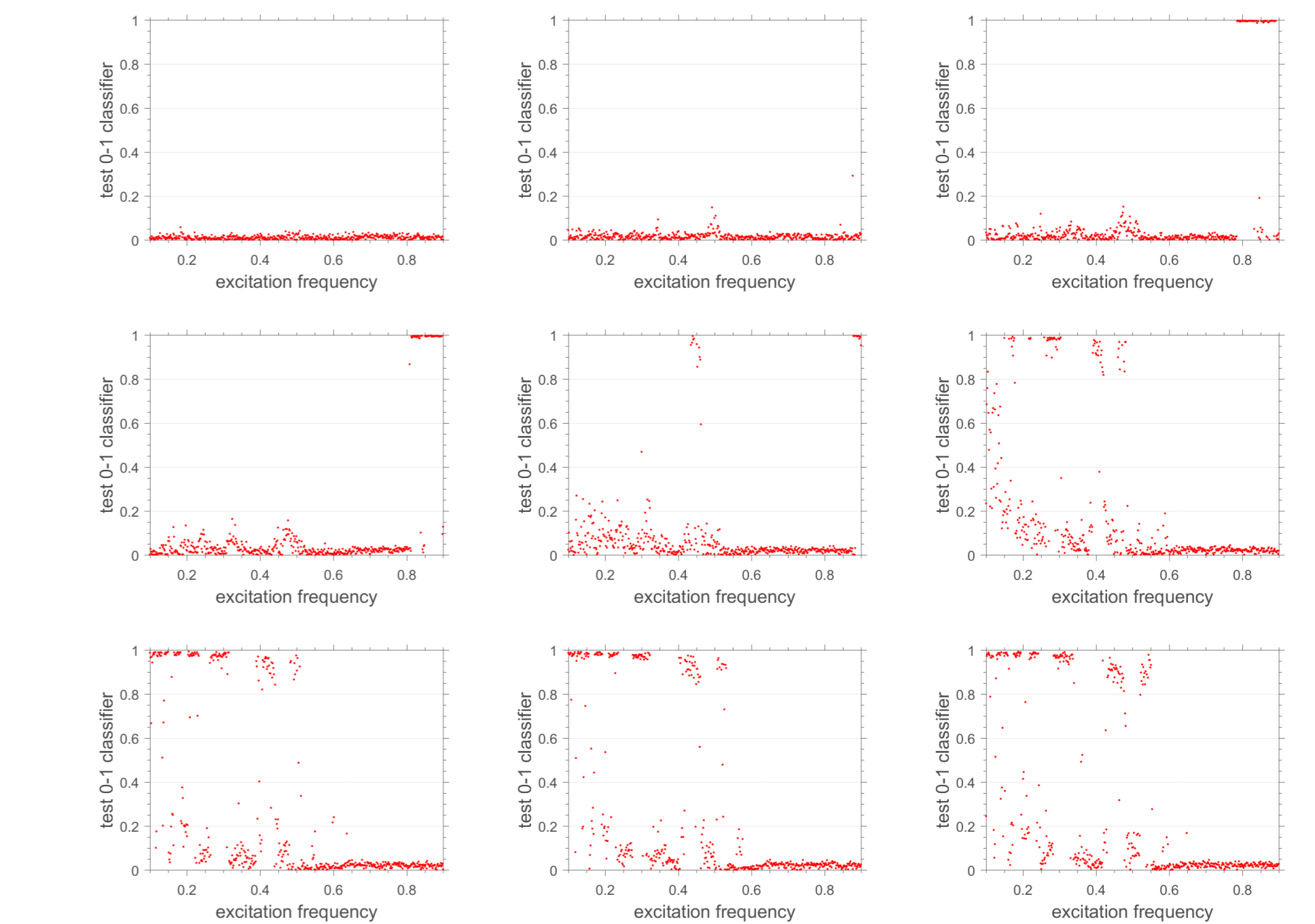
Relação entre a frequência de forçamento e o indicador do teste 0-1 para diferentes valores de amplitude de excitação f .
