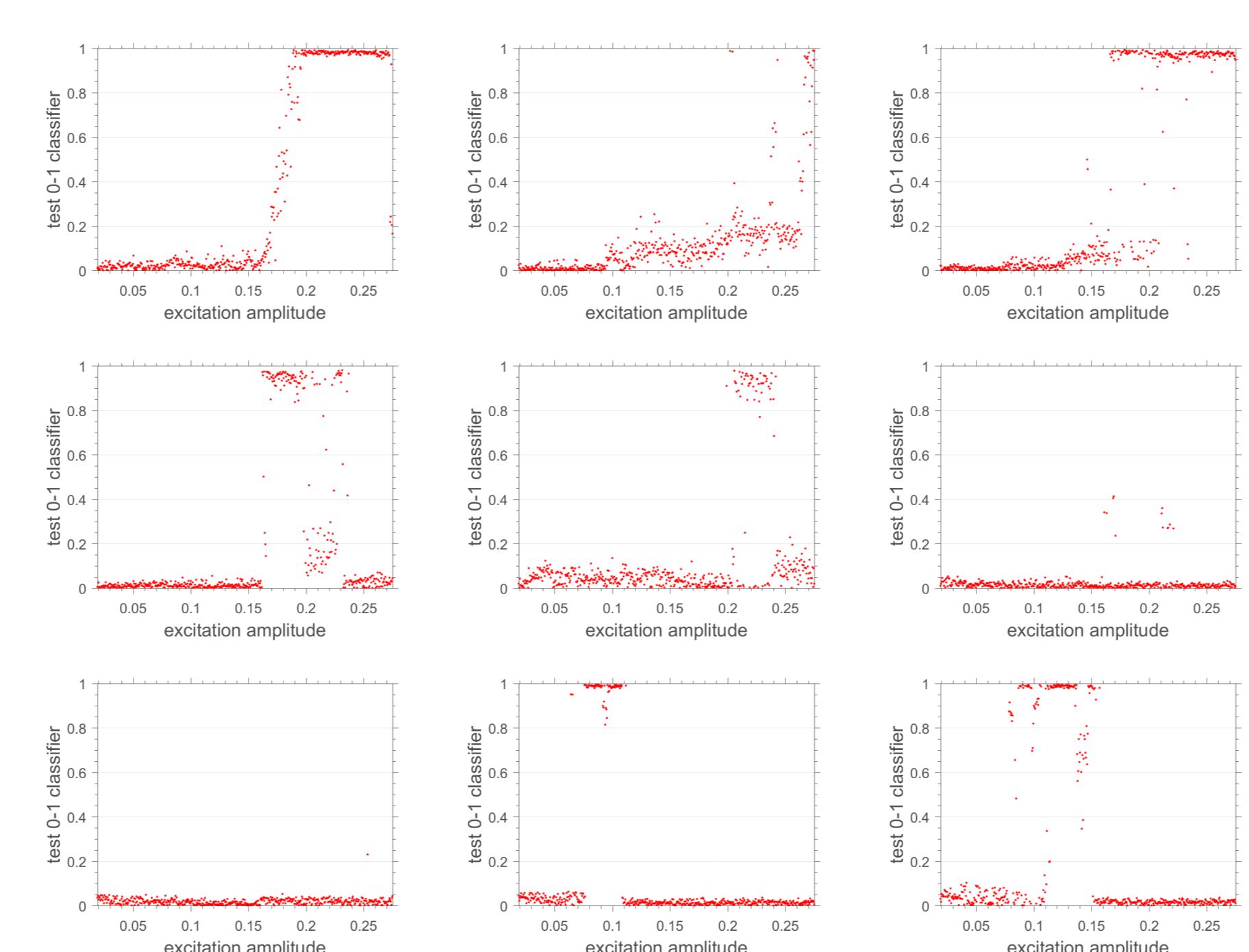
Relação entre a amplitude de forçamento e o indicador do teste 0-1 para diferentes valores de frequência de excitação \Omega .
