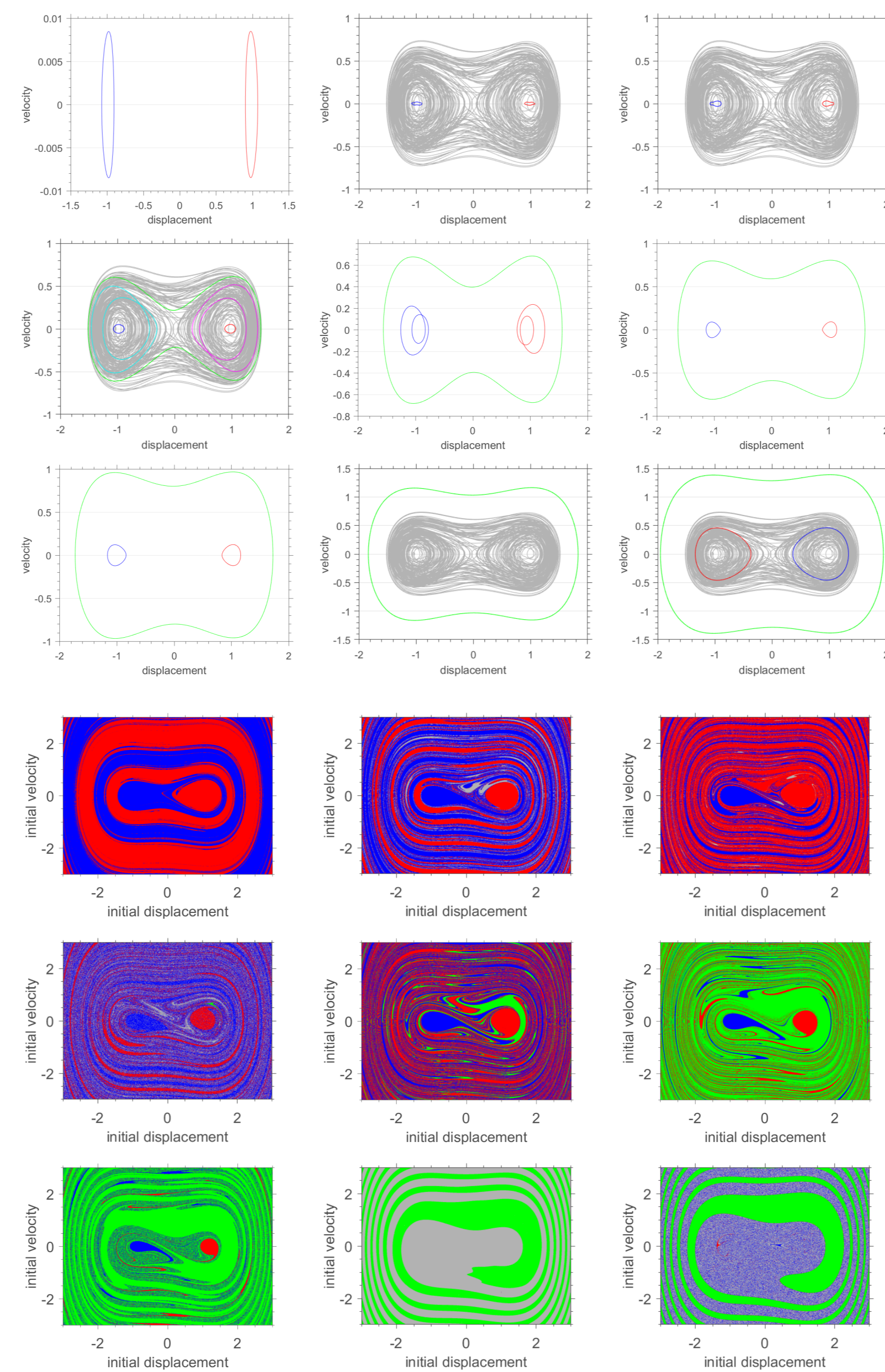
Atratores e bacias para f = 0.115 e 0.1 \leq \Omega \leq 0.9
