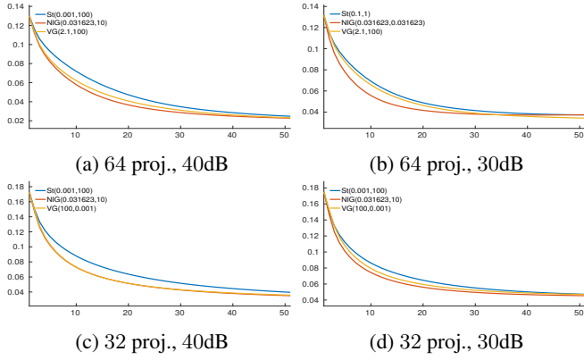
FIGURE 4 – Etude 2D : comportement des algorithmes JMAP pour les hyperparamètres optimaux, 40dB et 30dB.
