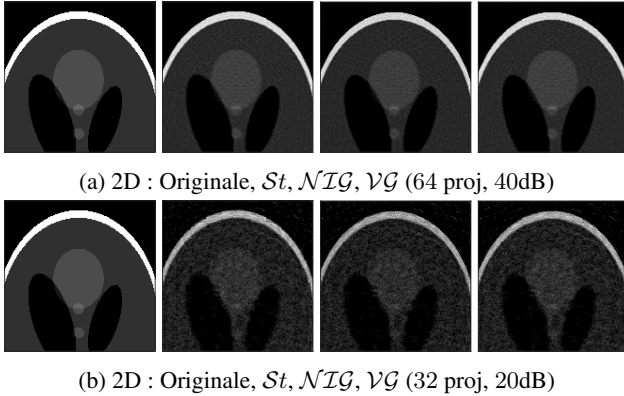
FIGURE 5 – Reconstructions 2D correspondant à St , \mathcal{NIG} et \mathcal{VG}
