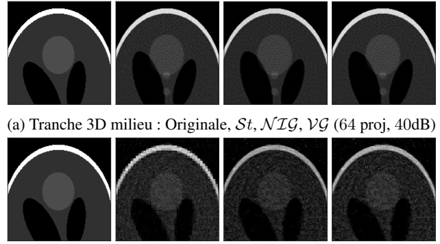
FIGURE 6 – Reconstructions 3D correspondant à St , \mathcal{NIG} et \mathcal{VG}
