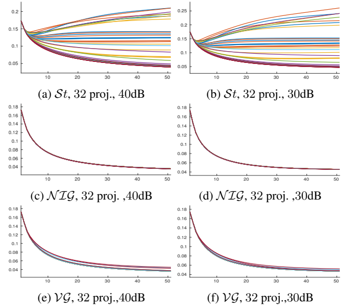
FIGURE 3 – Etude 2D : Performances de la reconstruction des algorithmes JMAP (NMSE) pendant les itérations en fonction des hyperparamètres.
