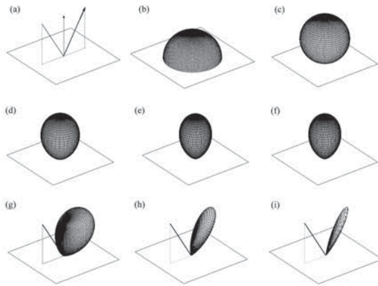
Fig. 2 : Exemples de lois de réflexion utilisées dans les simulations SPPS : (a) spéculaire, (b) uniforme, (c) Lambert (diffusion idéale), (d-f) lois en w^n ( n=2,3 et 4 ), (g-i) lois semi-diffuses
