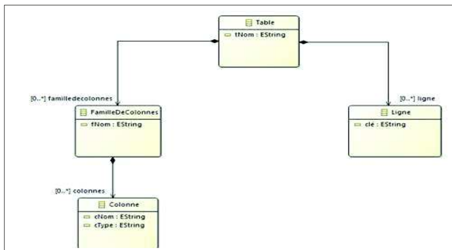
Figure 4. Méta-modèle cible
