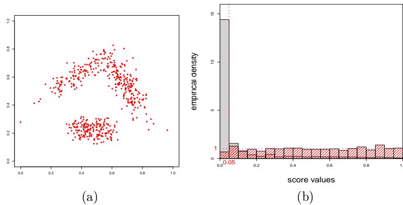
FIGURE 1 – (a) Echantillon nominal \mathcal{S} utilisé pour le calcul de \tau (b) Distribution des probabilités critiques (rouge : points nominaux - gris : points tirés selon une loi uniforme)
