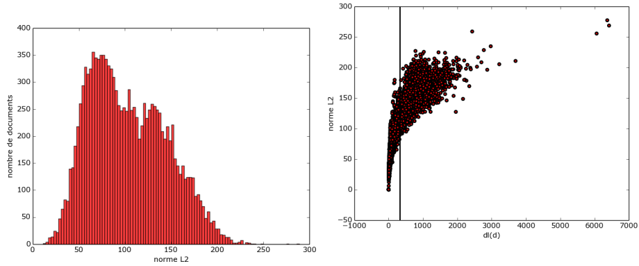
Figure 3. Norme L_2 des documents de la collection Tipster selon leur longueur dl(d) avec une pondération BM_{25+} (version modifiée selon (Lv et Zhai, 2011)); la ligne verticale représente la longueur moyenne ( avgdl ).
