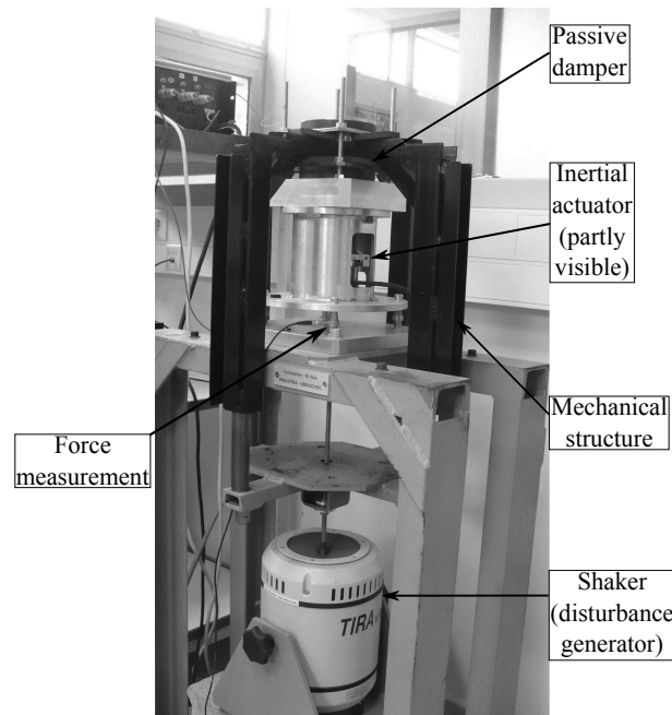
Figure 2. Le banc d'essai (photo).
