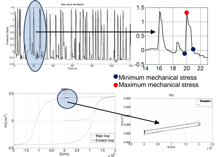
Figure 7: Comparaison mesure/simulation pour des cycles diélectriques d'extraction de l'énergie d'Ericsson.
