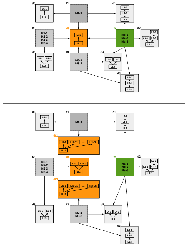
FIG. 1 – Le graphe multidimensionnel M_G initial (haut) et à la sortie de notre algorithme (bas)
