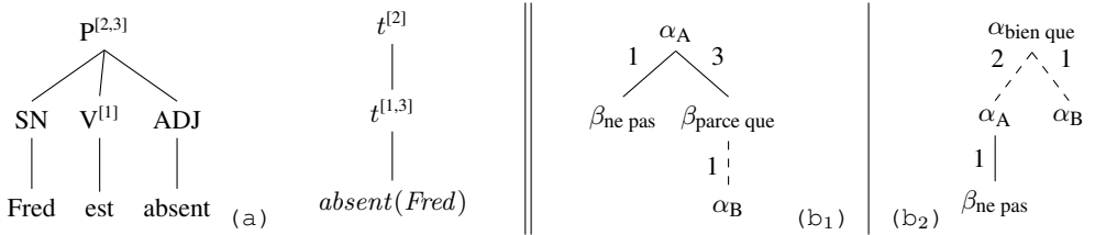
FIGURE 4 – Une structure phrastique (a), accompagnée des arbres de dérivations pour \neg A CONJ B avec une ConjC (b 1 ) ou une ConjP (b 2 ). Les liens [1] et [3] de \alpha_A étant situé au même nœud sémantique, l’arbre de gauche est une représentation sous-spécifiée qui, suivant l’ordre des adjonctions, conduit à deux arbres dérivés différents en sémantique mais un unique arbre pour la syntaxe.
