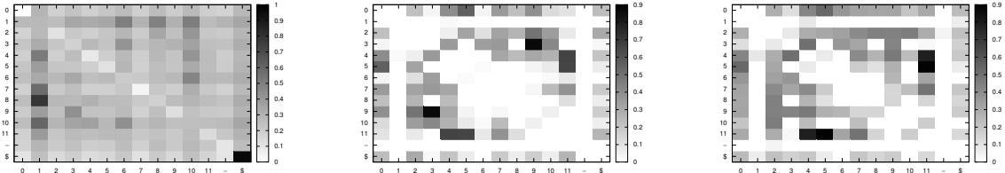
(a) SEDiL (Selkow).
