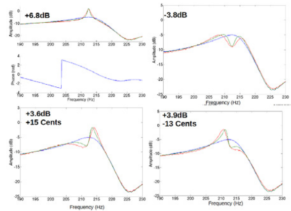
FIGURE 6 – Différents contrôles appliqués à la deuxième résonance de l'instrument, FT mesurées sans contrôle (bleu), avec contrôle (rouge) et simulation de contrôle (vert). Les contrôles sont tous réalisés avec G = 1 et Q = 50 , et quatre phases ciblées différentes. Haut-gauche : \phi_c = 0 . Haut-droite : \phi_c = \pi . Bas-gauche : \phi_c = \pi/2 . Bas-droite : \phi_c = 3\pi/2 .
