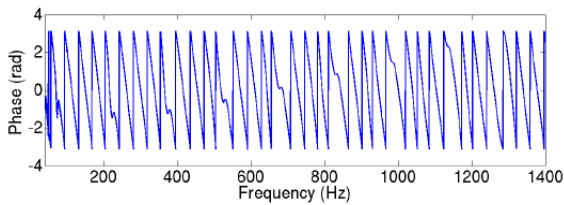
FIGURE 4 – Phase en boucle ouverte de la fonction de transfert du système.
