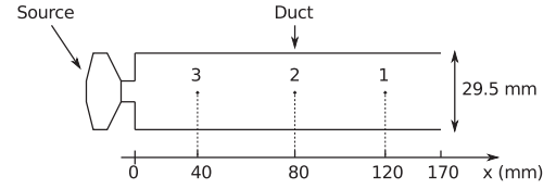
FIGURE 4 – Positions des points de mesures à l'intérieur de la maquette à un seul tube.
