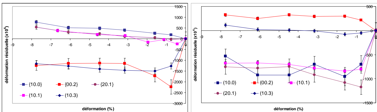
(a) (b) Figure 5 - Exemples d'évolution des déformations intergranulaires longitudinales (a) et transversales (b) en fonction de la déformation macroscopique pour différents plans cristallographiques.
