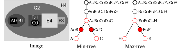
FIGURE 3 – Une image synthétique, son Min-tree (au milieu) et son Max-tree (à droite). Les régions critiques sont représentées par des cercles rouges : ce sont des nœuds ayant plus d’un enfant et les feuilles. Les TBMRs sont les régions correspondants aux nœuds remplis en rouge.
