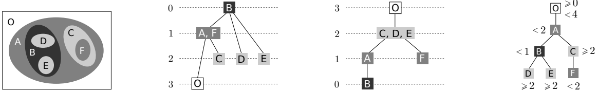
FIGURE 2 – Une image (à gauche), ses Max-tree et Min-tree (au milieu), et son arbre des formes (à droite).
