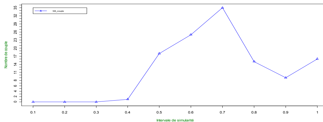
Figure 4 : Similarité Classe/Classe
