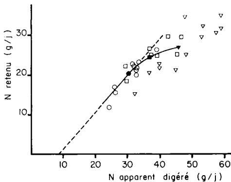
FIG. 1. — Relation entre l'azote apparemment digéré et l'azote retenu chez les veaux recevant les aliments : \circ , 15 ; \square , 17 ; \Delta , 21. La droite de régression ( NR = 0,907 NAD - 7,69 , R^2 = 0,83 ) représente la relation pour le régime 15, lorsque l'azote ingéré est limitant. \bullet , \blacksquare et \blacktriangle montrent les valeurs moyennes de l'azote retenu et de l'azote apparemment digéré.
