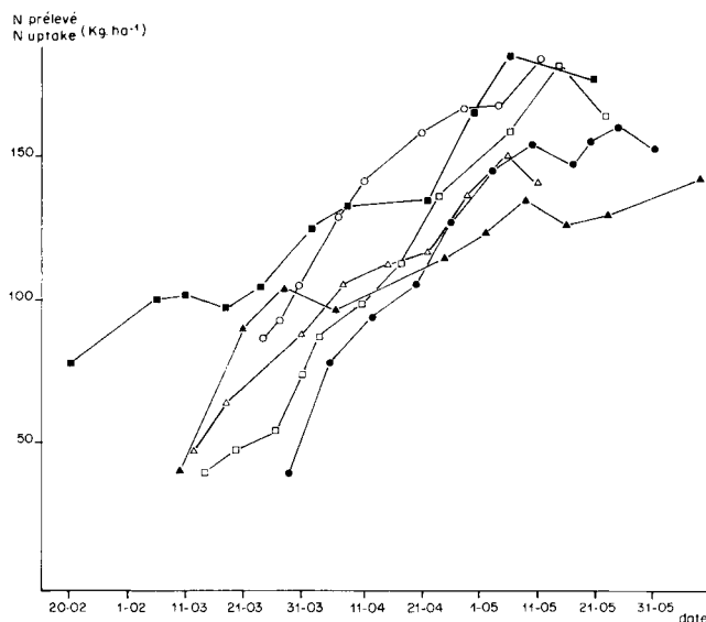
Figure 2 Prélèvements d'azote de la fétuque élevée « Ludelle » pour une nutrition azotée non limitante, au cours de la croissance de printemps (kg N. ha -1 ).
