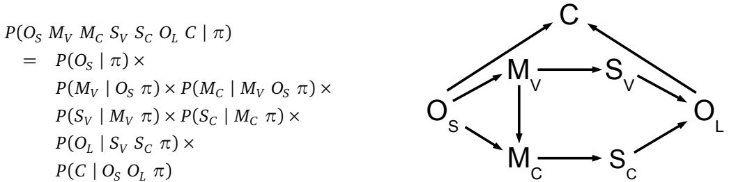
FIGURE 2: À gauche, la distribution de probabilité conjointe du modèle COSMO-Syllabes ; à droite, une représentation graphique de cette structure de dépendance probabiliste.
