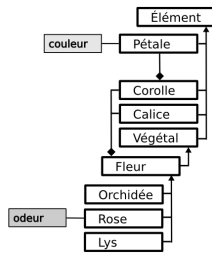
FIG. 1 – Exemple de deux ontologies o_1 et o_2 ; la subsomption est notée \blacktriangle , la méronymie \blacklozenge .
