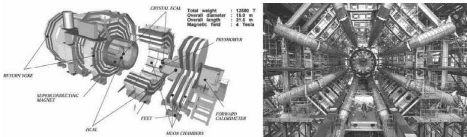
Fig. 3. Schéma écorché de CMS et photographie de sa cavité intérieure.
