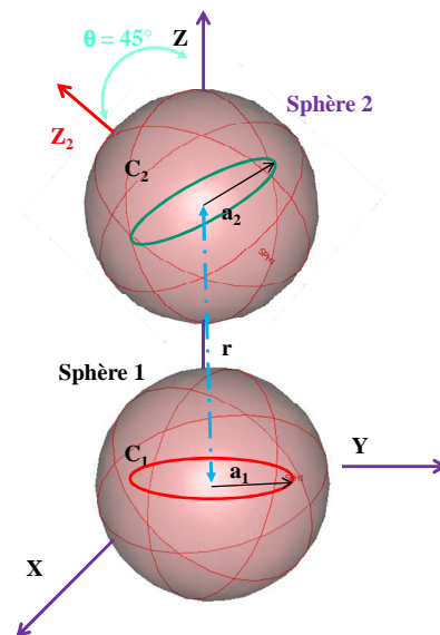
Fig.8 – Deux boucles de mêmes dimensions placées sur l'axe z où C_2 est à 45° du repère (x,y,z).
