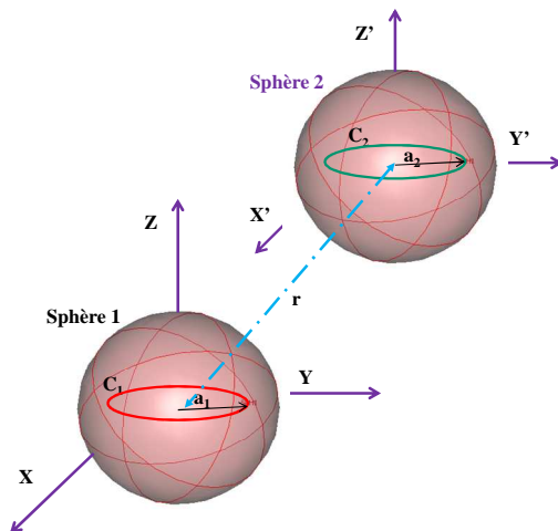
Fig.10 – Deux boucles qui ne se situent pas sur le même axe
