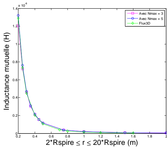
Fig.9 – Comparaison de l'inductance mutuelle entre deux boucles en fonction de la distance
