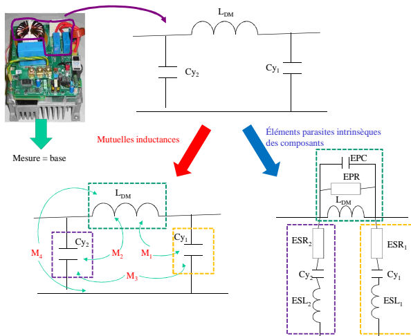
Fig.1 – Filtre avec éléments parasites.
