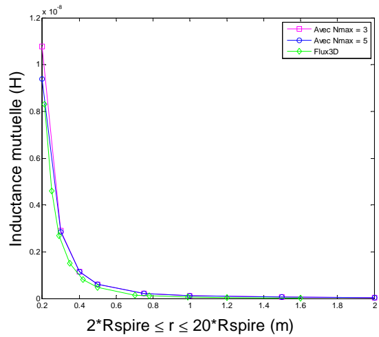
Fig.11 – Comparaison de l'inductance mutuelle entre deux boucles pas sur le même axe en fonction de la distance
