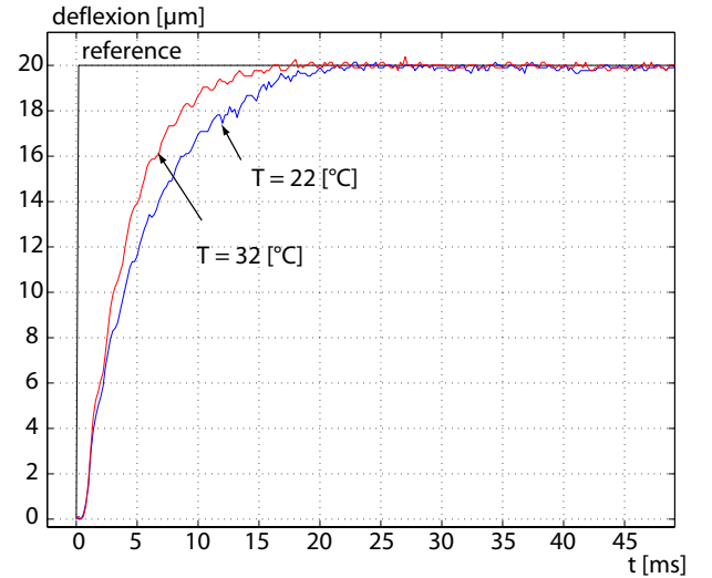
Fig. 13. Step response.
