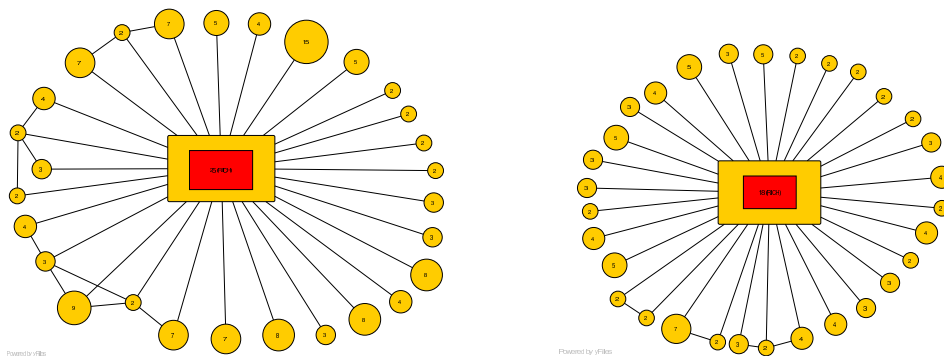
FIG. 2 – Graphe des communautés de G_{av} (à gauche) et G_{ap} (à droite). Les disques représentent les k -communautés extraites et le rectangle le reste des sommets (dont le club-huppé).
