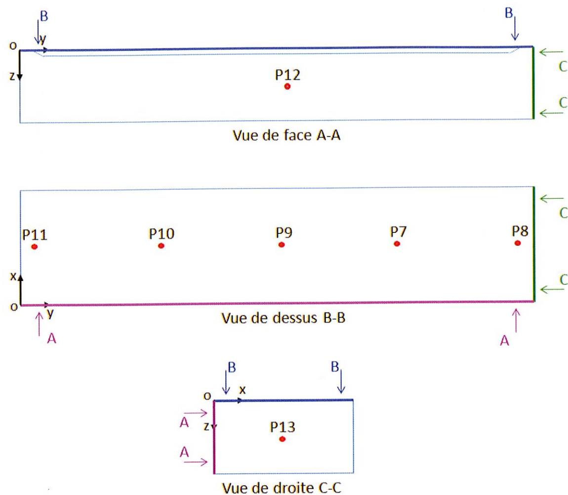
figure 6 Emplacement des capteurs de déplacement.
