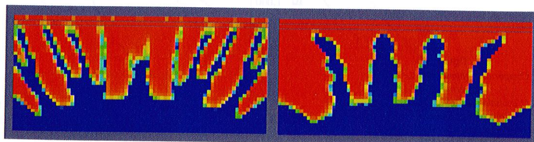
figure 21 Cartographies d'endommagement 2D dans la partie centrale de la poutre (1 600 mm) obtenues par les modèles de Mazars (gauche) et Ricrag (droite) pour une flèche de 14 mm.
