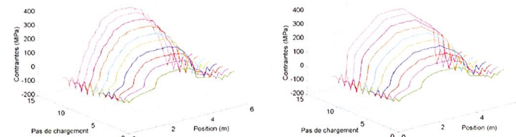
figure 23 Courbes de contraintes dans l'acier supérieur HA32 le plus proche de la surface en fonction de la position le long de l'acier et du pas de chargement [Modèles de Mazars (gauche) et Ricrag (droite)].
