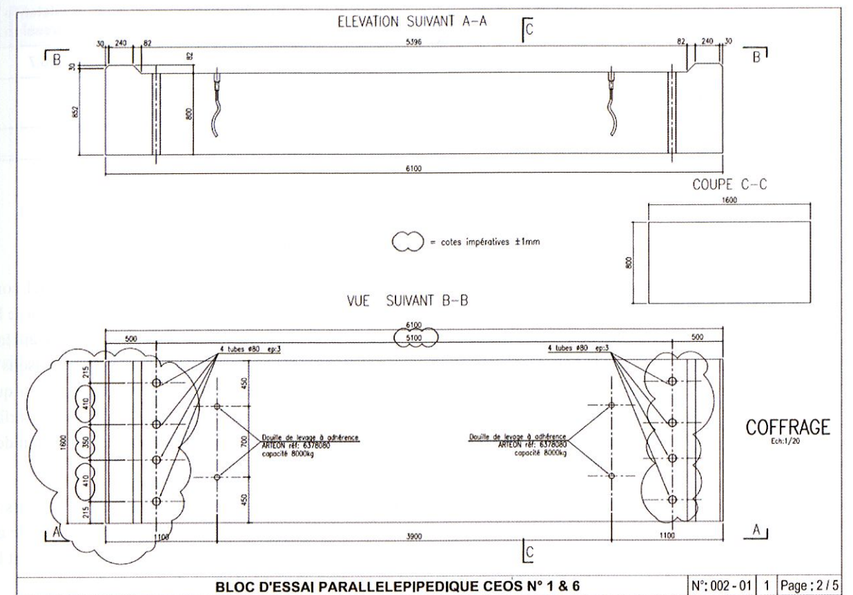
figure 1 Géométrie de la poutre.
