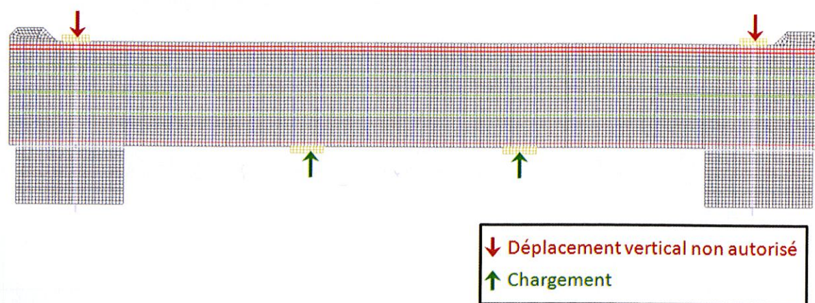
figure 11 Conditions aux limites du modèle 2D.
