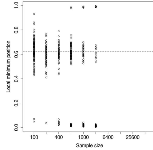
(d) Estimator related to \hat{f}_P
