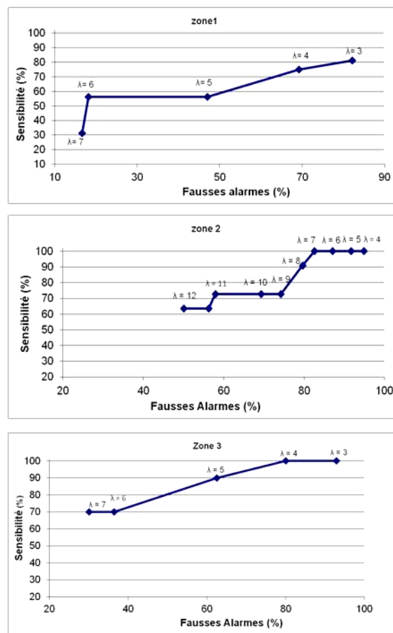
Figure 12 : Résultats de la sensibilité en fonction des fausses alarmes pour les zones 1, 2 et 3
