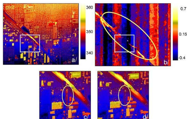
Figure 6: a: carte d'altitudes calculée par géométrie faisceau 2D, parallaxe 1 (en mètres). Les bandes verticales sont dues aux erreurs liées au calcul du capteur parfait. b: carte d'altitudes calculées par géométrie faisceau 2D parallaxe 2 (en pixel). c et d: cartes des altitudes calculées respectivement par géométrie faisceau 1D et par géométrie 2D (en mètres). L'ellipse montre une route d'altitude surestimée par la recherche 1D.
