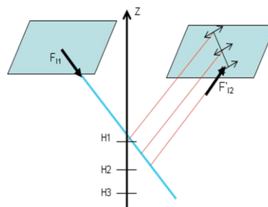
Figure 3: Recherche bidimensionnelle des pixels homologues
