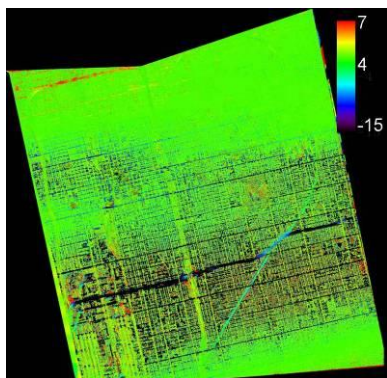
Figure 5 : Différence entre les cartes d'altitudes obtenues avec une mise en correspondance 2D et 1D (échelle en mètres)
