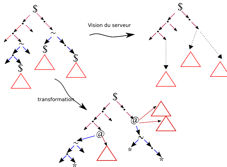
Figure 1: Exemple d'arbre Hop
