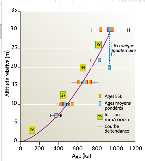
▲ Fig. 3 : Distribution des âges ESR obtenus en fonction de l'altitude relative de différents témoins de nappes alluviales fossiles échantillonnés dans la vallée du Cher en aval de Vierzon. Des vitesses d'incision moyennes en sont déduites.
