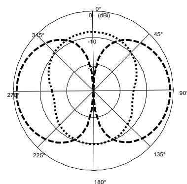
(d) DC voltage : 1.5V, f = 620 MHz (...) E_{\phi} and E_{\theta} (--) in XZ plane
