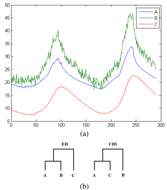
FIGURE 1 – (a) Trois séries temporelles A, B et C. (b) Classification hiérarchique des séries temporelles A, B et C basée sur les distances ED et CID.
