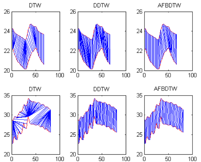
FIGURE 4 – Comparaison visuelle des performances des trois méthodes de mise en correspondance avec la DTW, DDTW et AFBDTW
