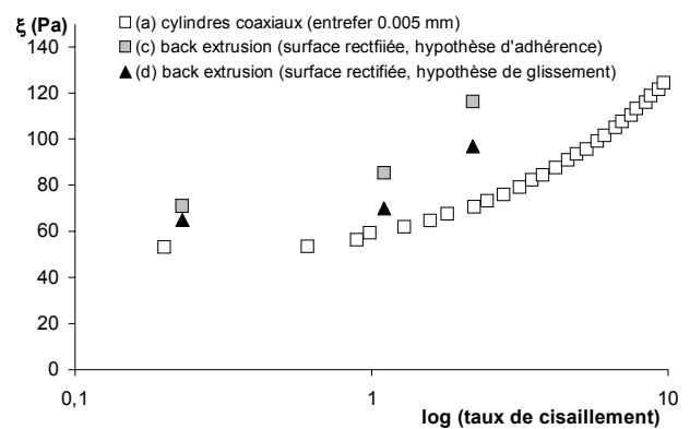
Fig. 9 : comparaison de rhéogrammes obtenus pour le mélange huile /sucre : (a) par cylindres coaxiaux, (d) par back-extrusion parois striées, (c) back-extrusion parois lisses, dépouillée en faisant l'hypothèse d'un champ de vitesse adhérent
