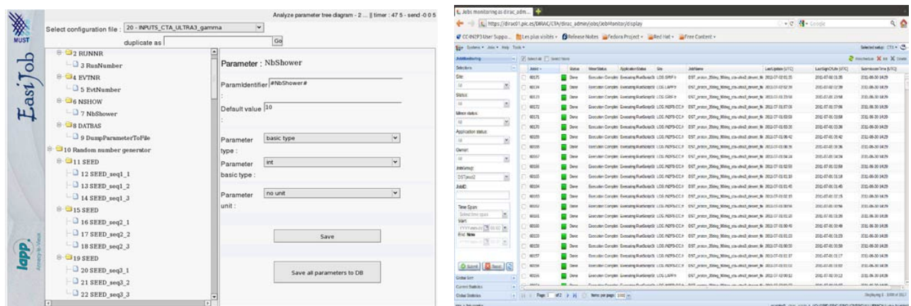
Figure 4.1: Interface web d'une des applications EasiJob développée pour CTA: sélection de la configuration du logiciel des simulations Monte Carlo et son interface de soumission ( Web interface of one of the EasiJob applications developed for CTA: software and workflow configuration interface selection for Monte Carlo simulations submitted to the Grid ). Figure 4.2: Service web basé sur le système DIRAC et développé pour CTA pour l'accès et l'interface aux jobs d'analyse et leurs résultats ( Web service based on DIRAC and developed for CTA devoted to user data access and interface to data analysis jobs on the Grid ).
