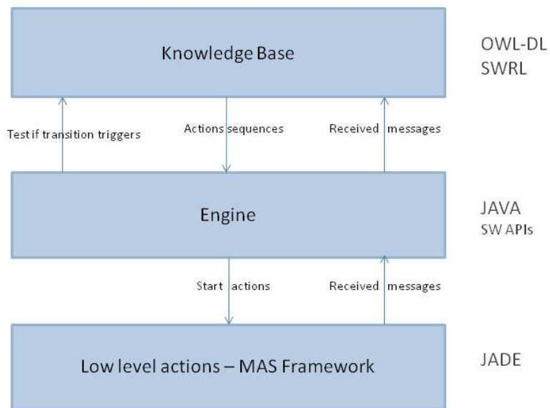
Fig. 1.1 : SAM Agent architecture
