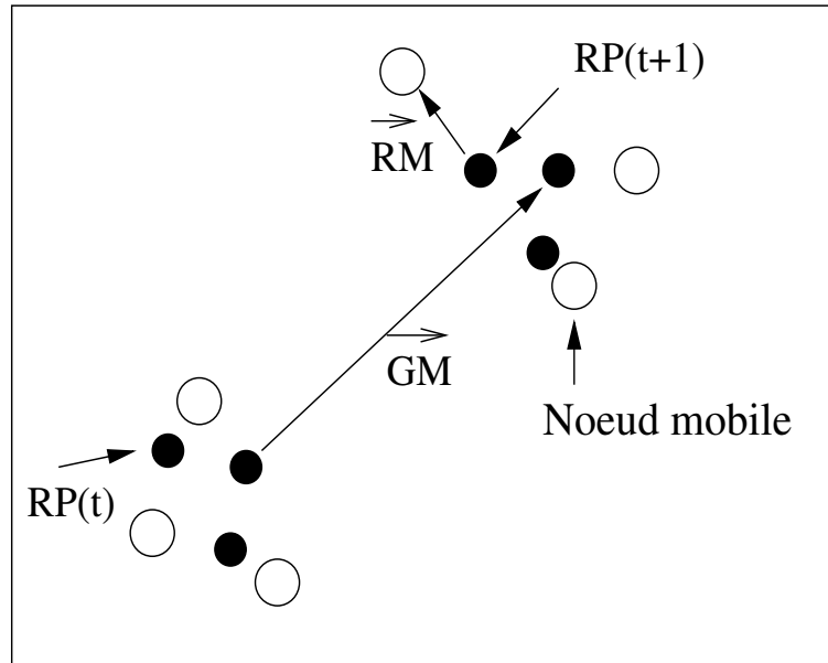
FIG. 4.11 – Mouvements de 3 nœuds utilisant le modèle RPGM
