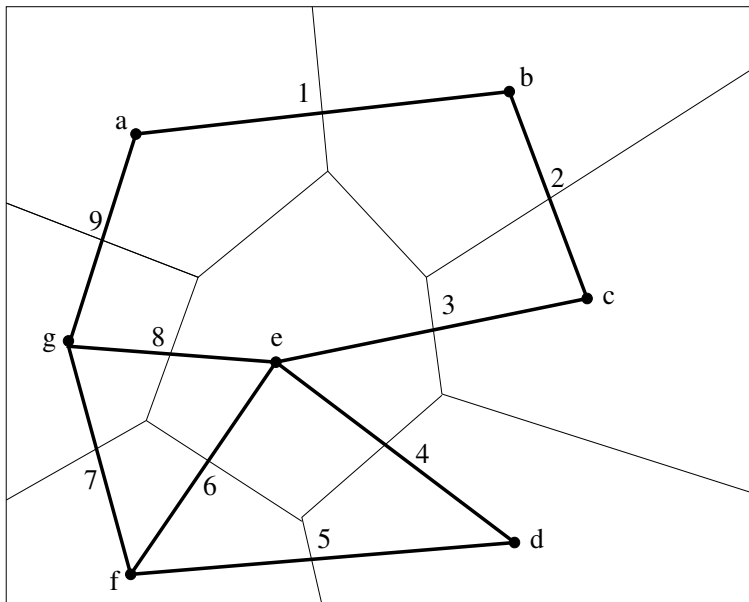
FIG. 7.15 – Graphe numéroté
