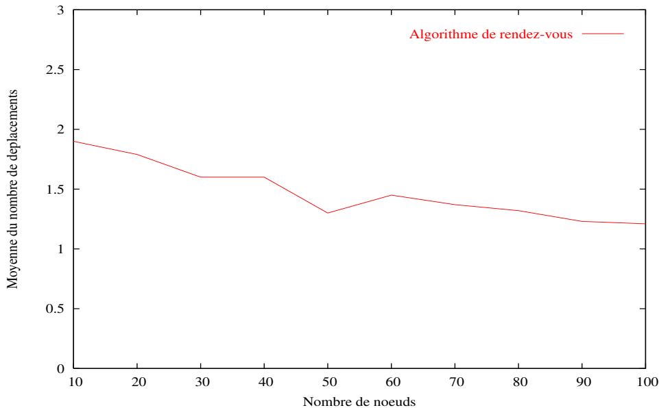
FIG. 9.3 – Le nombre de déplacements par rapport au nombre de nœuds
