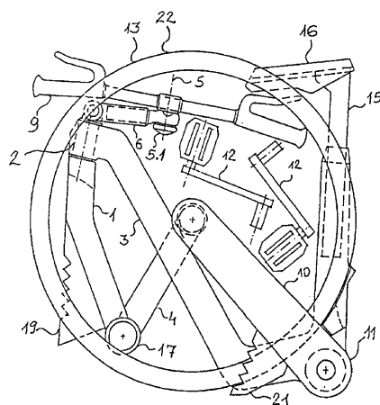
Une fois replié, ce vélo coréen consomme une place très réduite. Brevet déposé en 2001, KR100792059B1.
