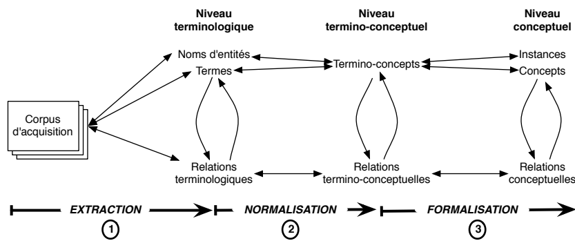
FIGURE 1: Les trois niveaux de connaissance et les trois étapes de la méthodologie de TERMINAE
