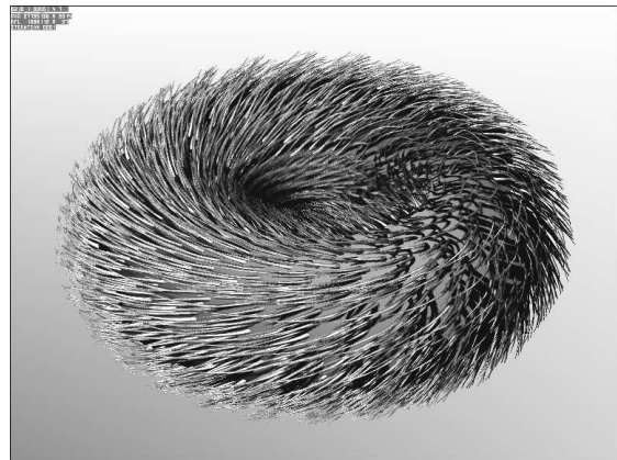
FIG. 10 - à gauche : poils dessinés cycliquement dans un volume 128x128x128 (compressé à 93%). Le rendu du texel seul prend 3.5 minutes. à droite : plaquage sur un tore composé de 240 patches bilinéaires (12 minutes).
