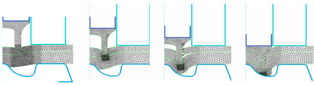
Figure 4 - Modélisation du procédé de rivetage autopoinçonneur en configuration 2D axisymétrique.
