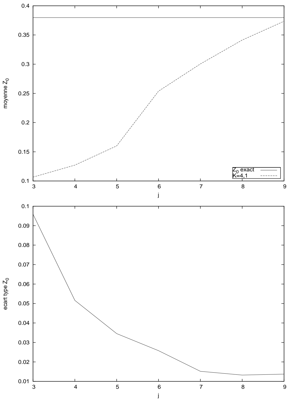
FIG. 6.2 – Convergence de Z_0 pour une grille de discrétisation non uniforme, \alpha = 0,5 et K = 4,1 .
