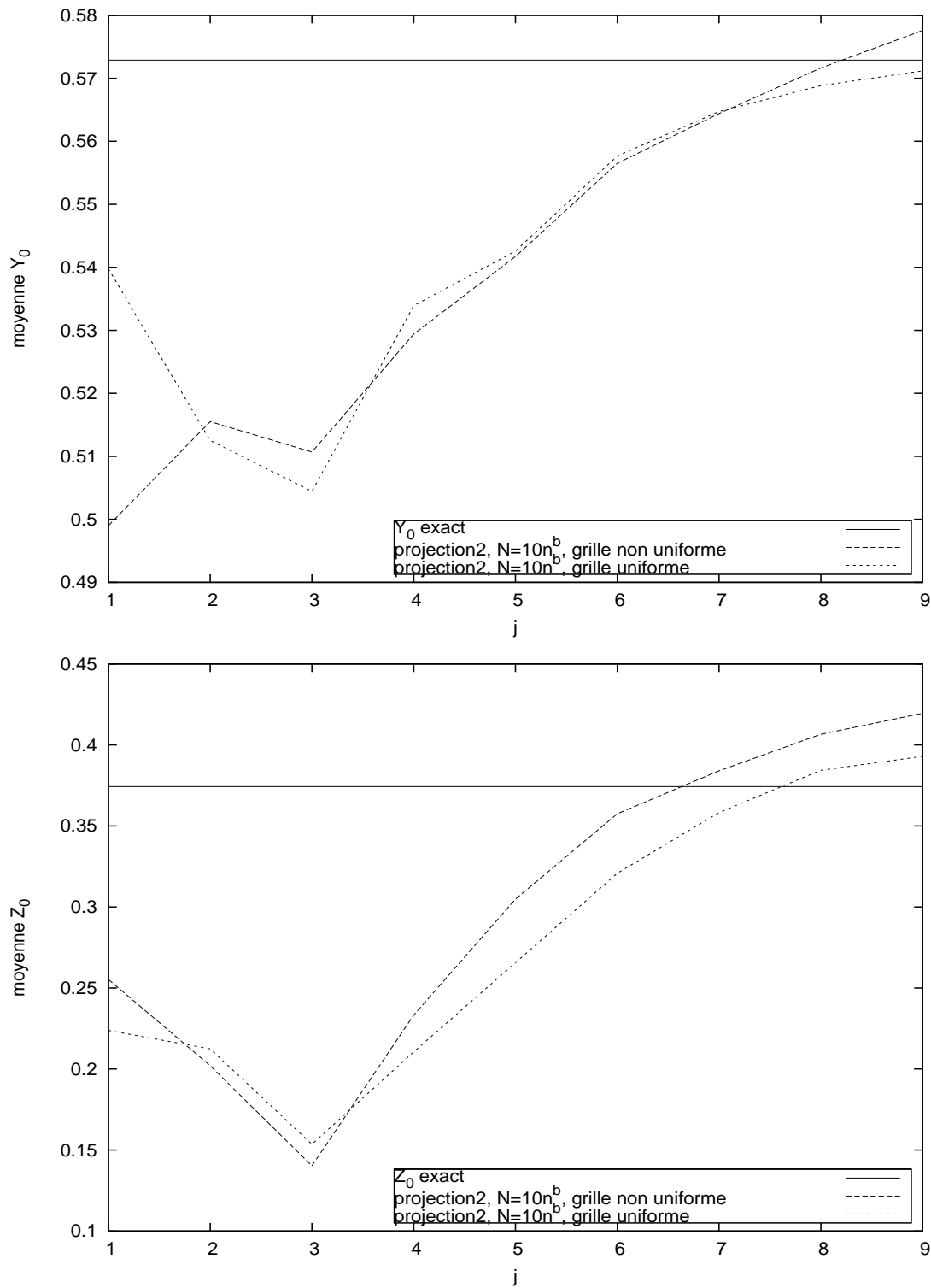
FIG. 6.11 – Convergence de Y_0 et de Z_0 lorsque \alpha = 0, 1 .
