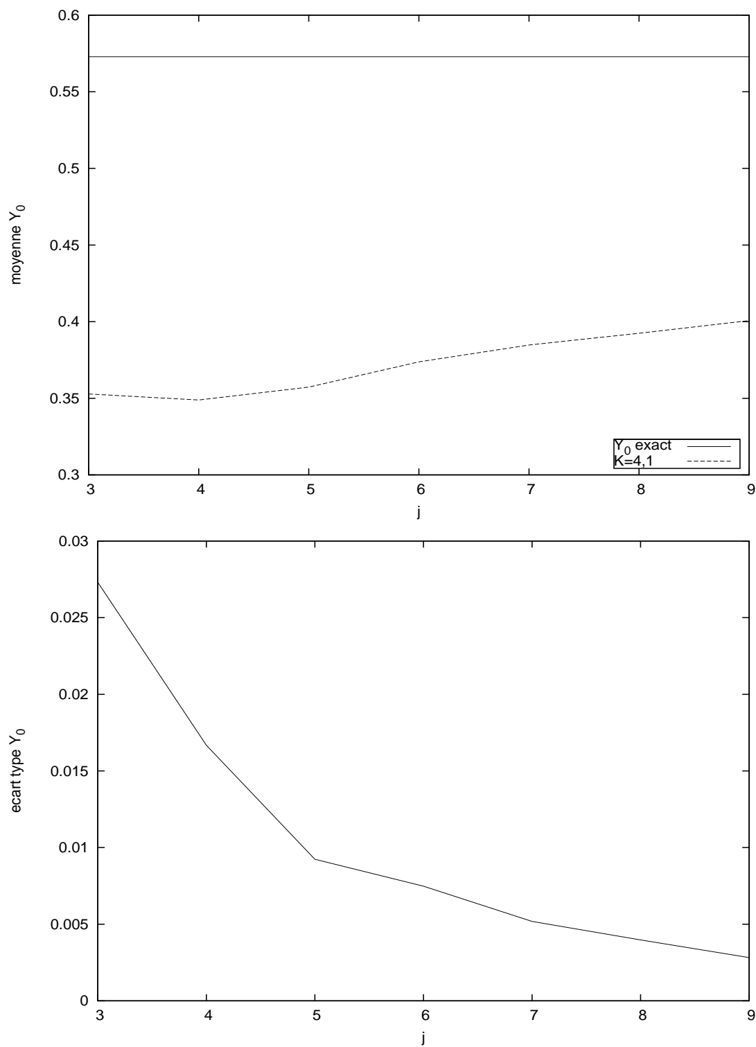
FIG. 6.3 – Convergence de Y_0 pour une grille de discrétisation non uniforme, \alpha = 0, 1 et K = 4, 1 .
