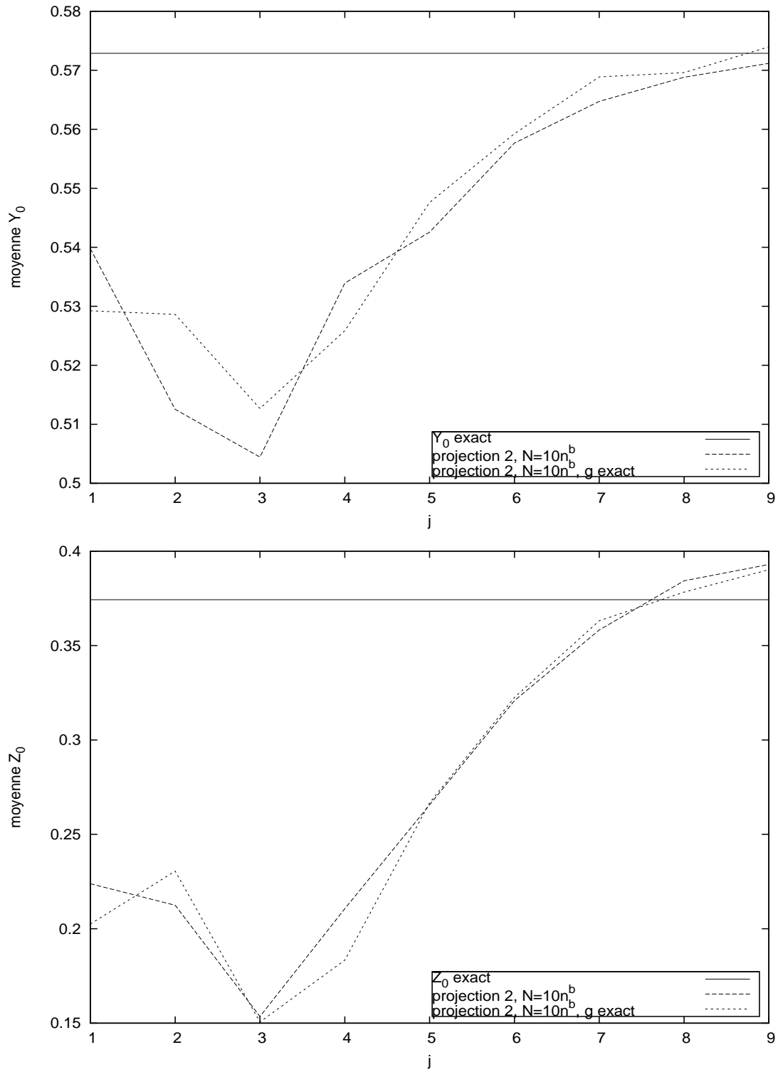
FIG. 6.13 – Convergence de Y_0 et de Z_0 lorsque la condition terminale g n'est pas approchée ( \alpha = 0, 1 ).
