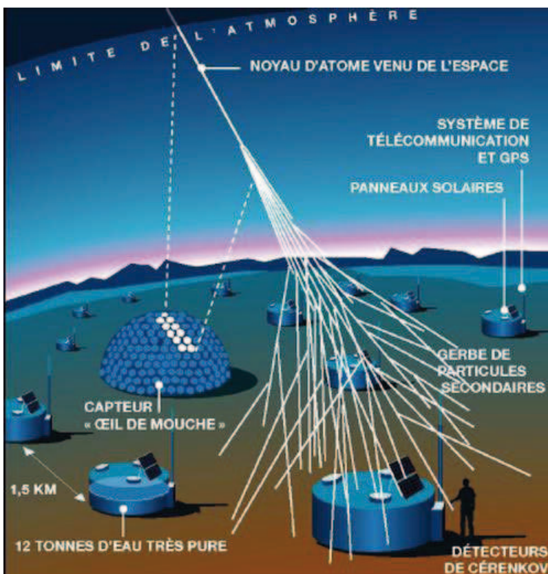
FIGURE 2.1: Schéma de l'Observatoire Pierre Auger
