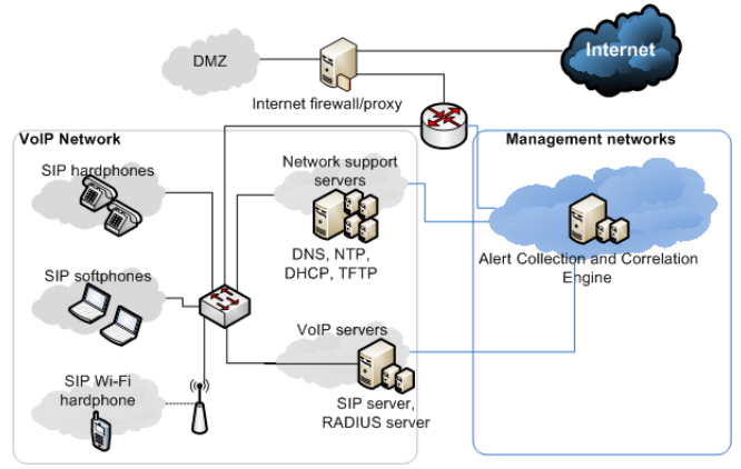
Fig. 4. The VoIP testbed
